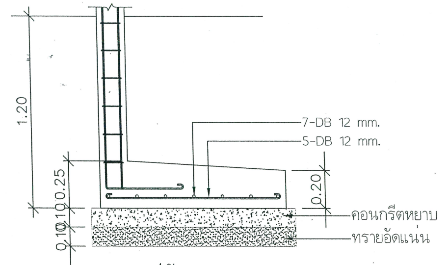
รูปตัด F มาตรา 1 : 25
