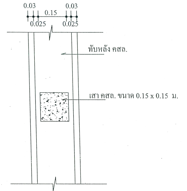
รูปตัด ข - ข มาตราส่วน 1 : 10
