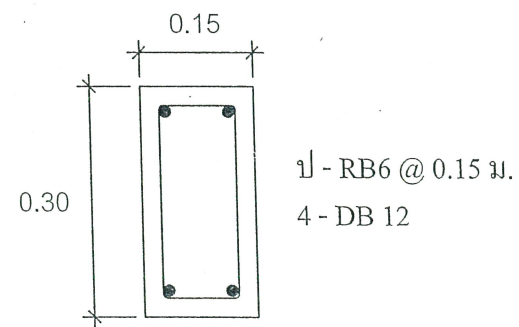
ขยายคานคอดิน GB1 มาตราส่วน 1 : 10
