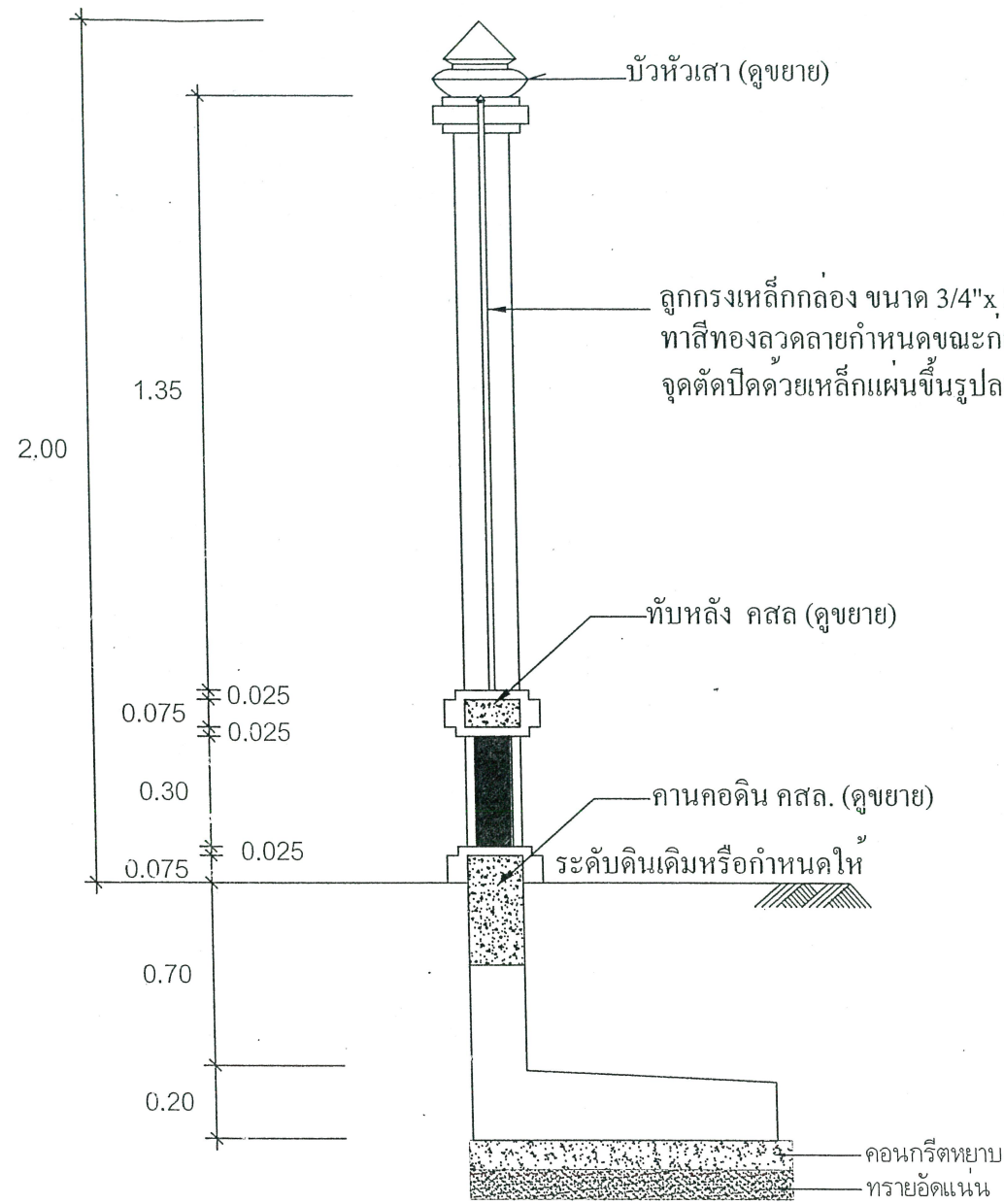
รูปตัด ก - ก มาตราส่วน 1 : 20
