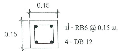
ขยายเสา C1 มาตราส่วน 1 : 10
